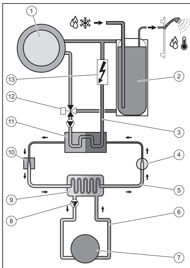
1 Varmeanlegg
